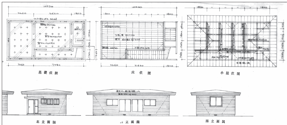
1973年竣工の初代自治会館の設計図面 (提供: 北沢建設株式会社)
